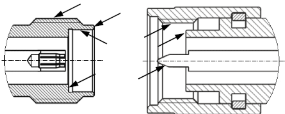
Рисунок 4 – Соединители тип 2,4 мм, 2,92 мм, 3,5 мм и IX (розетка и вилка)
