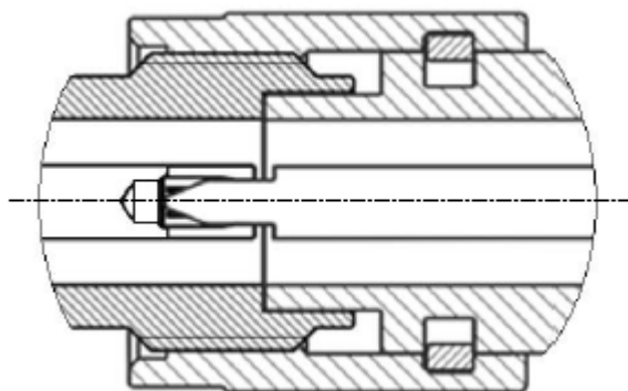
Рисунок 8 – Соединители тип 2,4 мм, 2,92 мм, 3,5 мм и IX (розетка слева, вилка справа)
