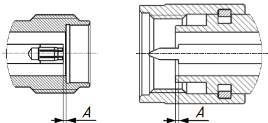
Рисунок 6 – Соединители тип 2,4 мм, 2,92 мм, 3,5 мм и IX (розетка и вилка)
