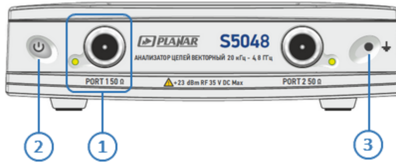
Рисунок 11 – Передняя панель
