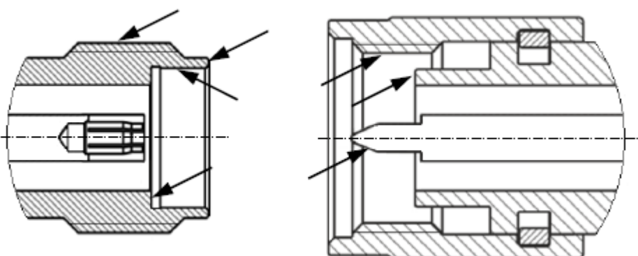
Рисунок 7 – Соединители тип 2,4 мм, 3,5 мм и IX (розетка и вилка)
