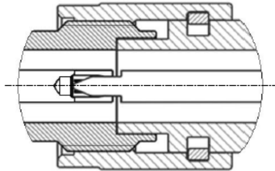
Рисунок 11 – Соединители тип 2,4 мм, 3,5 мм и IX (розетка слева, вилка справа)
