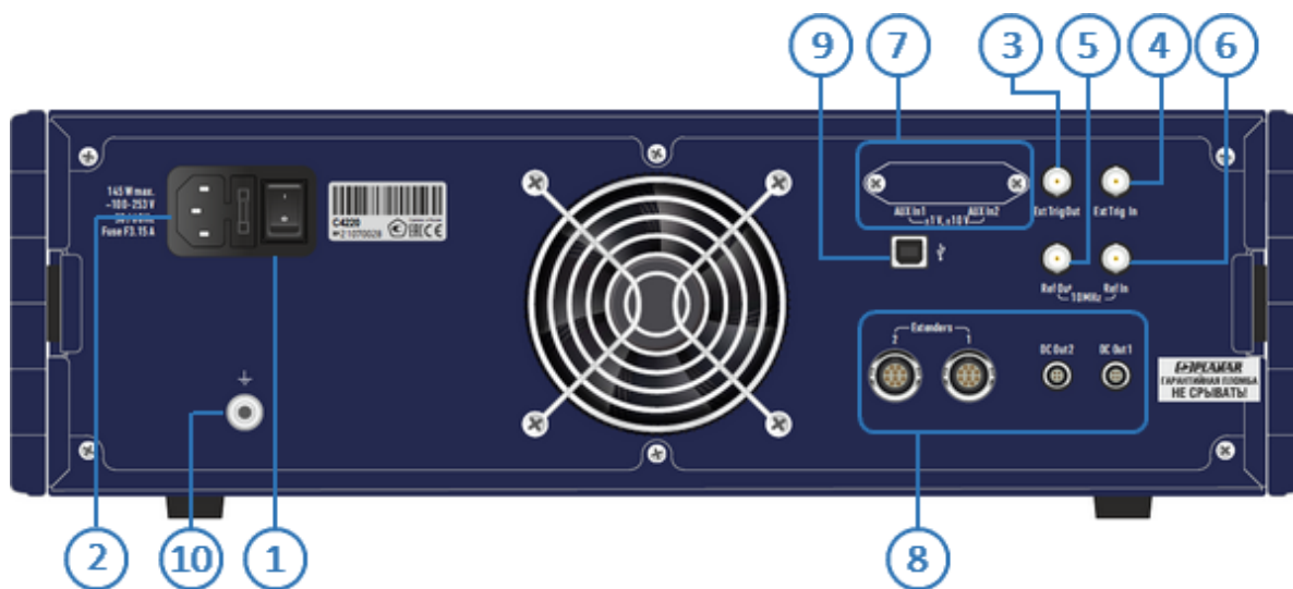
Рисунок 37 – Задняя панель
