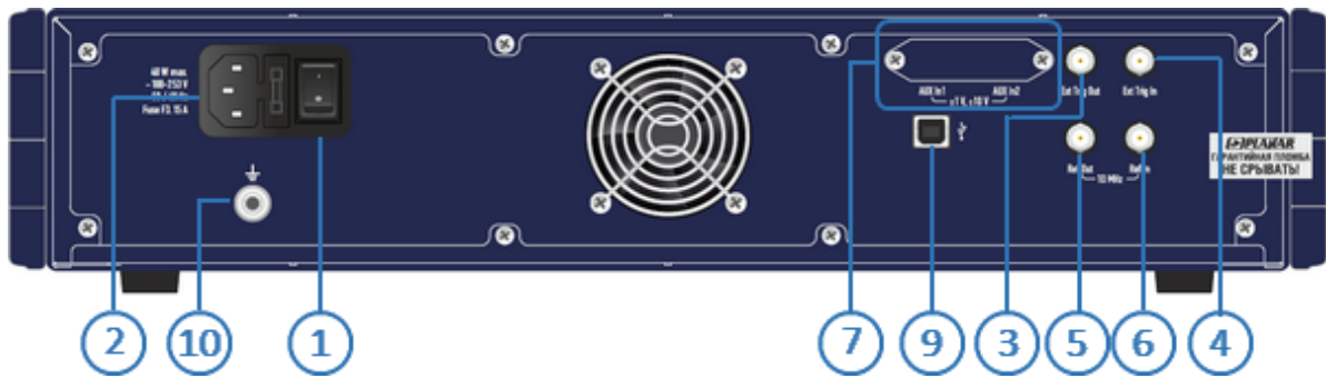
Рисунок 23 – Задняя панель
