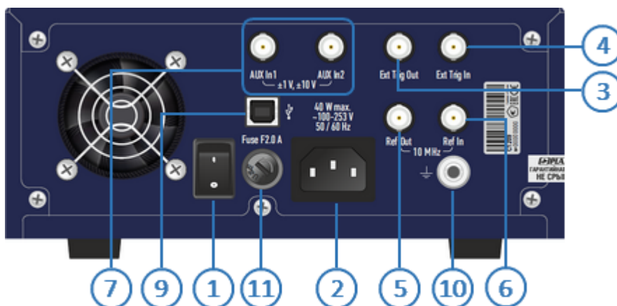
Рисунок 13 — Задняя панель
