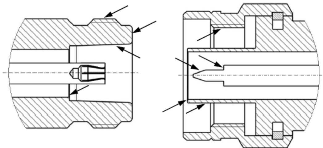
Рисунок 35 – Соединители типа N и III (вилка и розетка)
