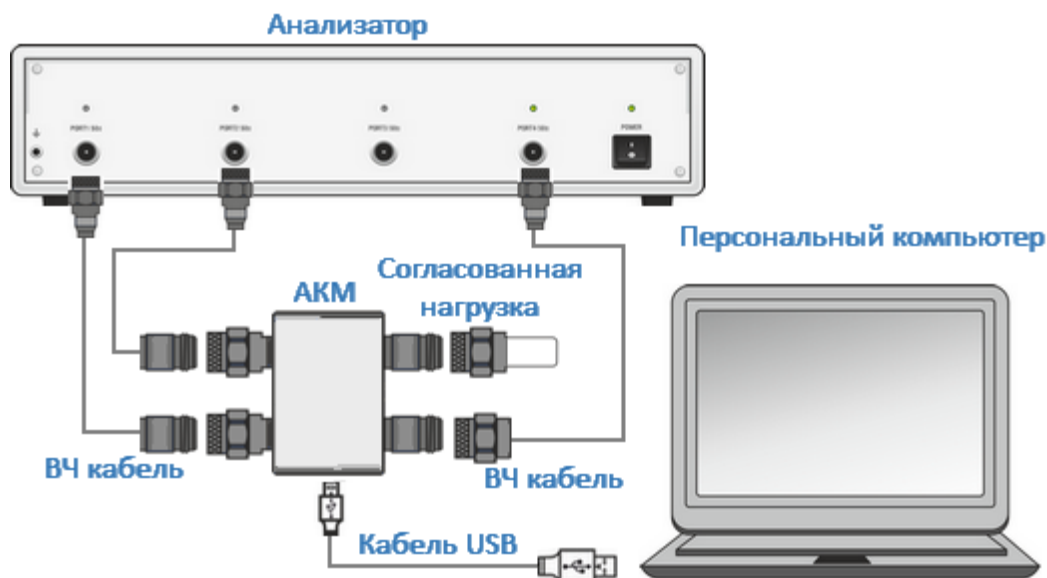
Рисунок 30 – Схема включения модуля для выполнения полной трехпортовой калибровки
