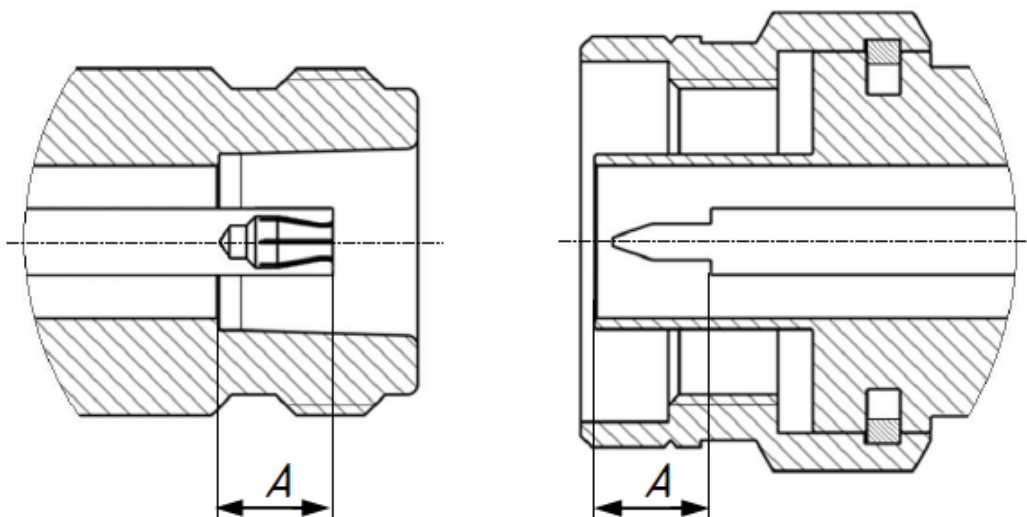
Рисунок 37 – Соединители типа N и III (розетка, вилка)
