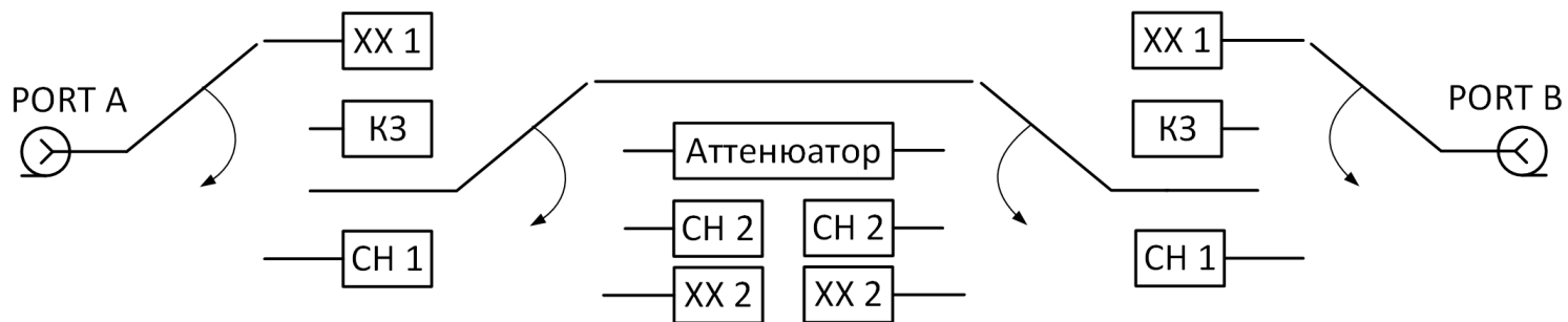
Рисунок 2 – Функциональная схема ACM2526, ACM2532, ACM2544, ACM8000T
