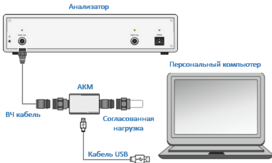
Рисунок 27 – Схема включения модуля для выполнения полной однопортовой калибровки
