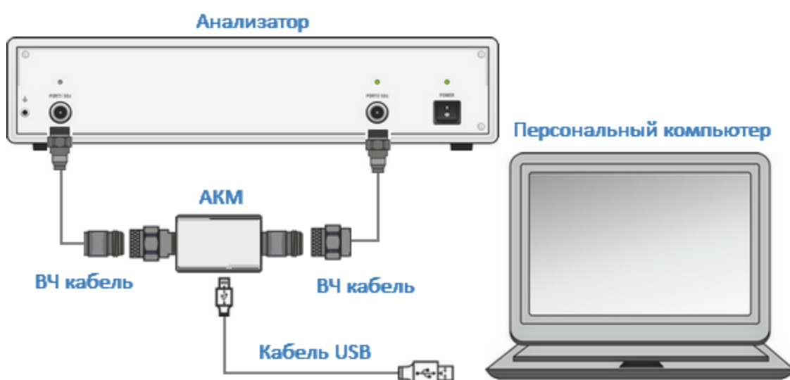
Рисунок 28 – Схема включения модуля для выполнения однонаправленной двухпортовой калибровки
