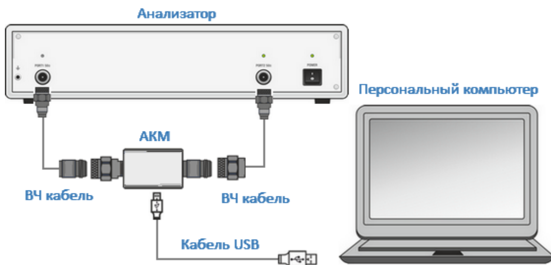
Рисунок 29 – Схема включения модуля для выполнения полной двухпортовой калибровки
