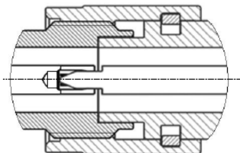
Рисунок 40 – Соединители типа 2,4 мм, 2,92 мм, 3,5 мм, IX (справа вилка, слева розетка)
