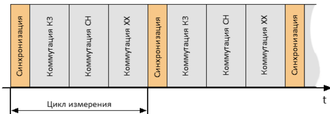
Рисунок 7 – Цикл измерения
