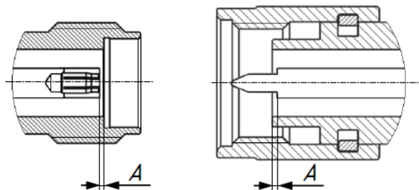
Рисунок 38 – Соединители 2,4 мм, 2,92 мм, 3,5 мм, IX (розетка, вилка)
