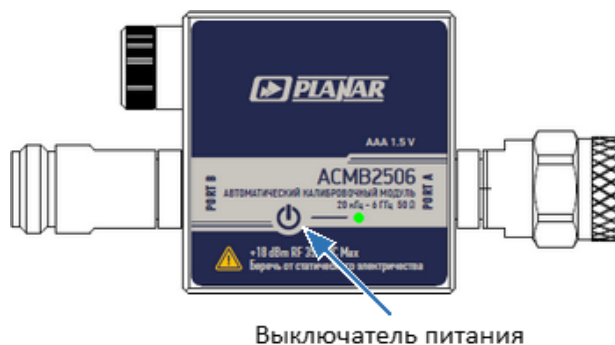
Рисунок 23 – Выключатель питания
