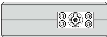
2,4 мм и 2,92 мм, розетка
