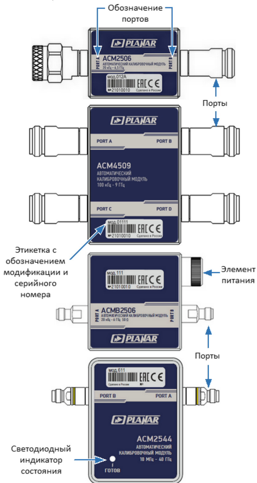
Рисунок 9 – Основные элементы модулей
