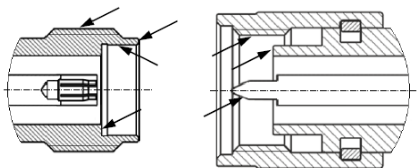
Рисунок 36 – Соединители 2,4 мм, 2,92 мм, 3,5 мм, IX (розетка и вилка)
