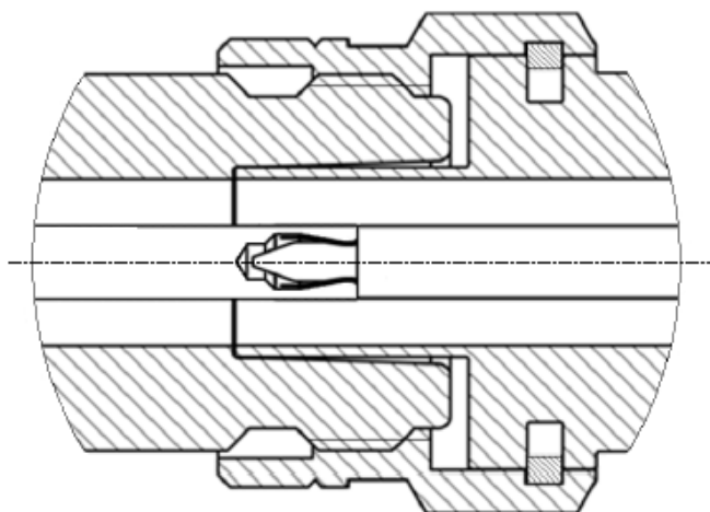
Рисунок 39 – Соединители типа N и III (справа вилка, слева розетка)
