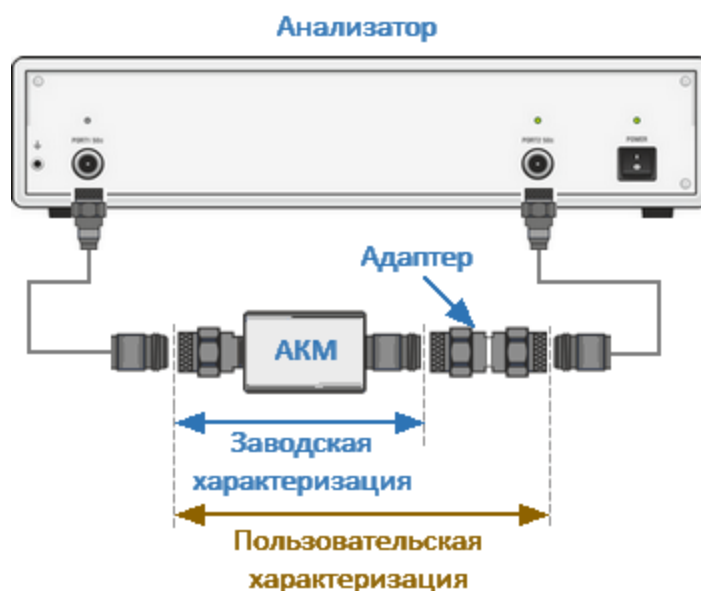
Рисунок 32 – Заводская и пользовательская характеристики
