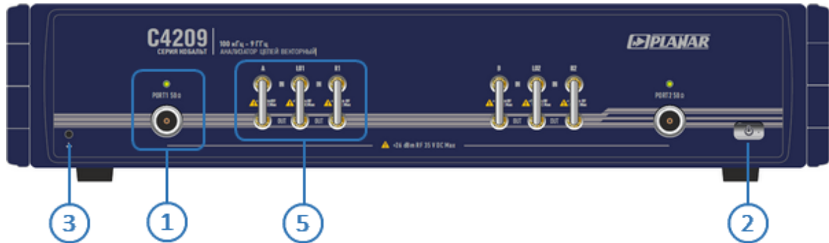
Рисунок 30 – Передняя панель
