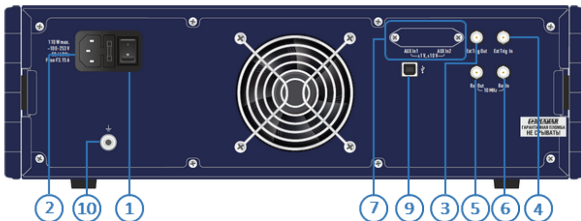
Рисунок 39 – Задняя панель
