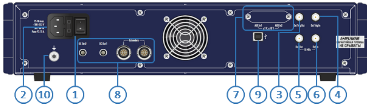
Рисунок 31 – Задняя панель
