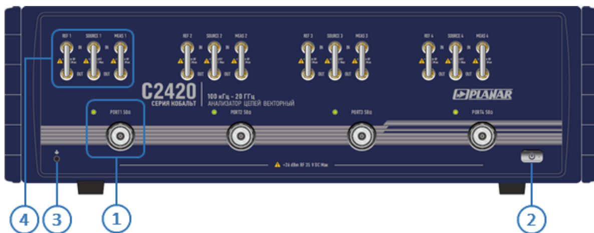
Рисунок 38 – Передняя панель
