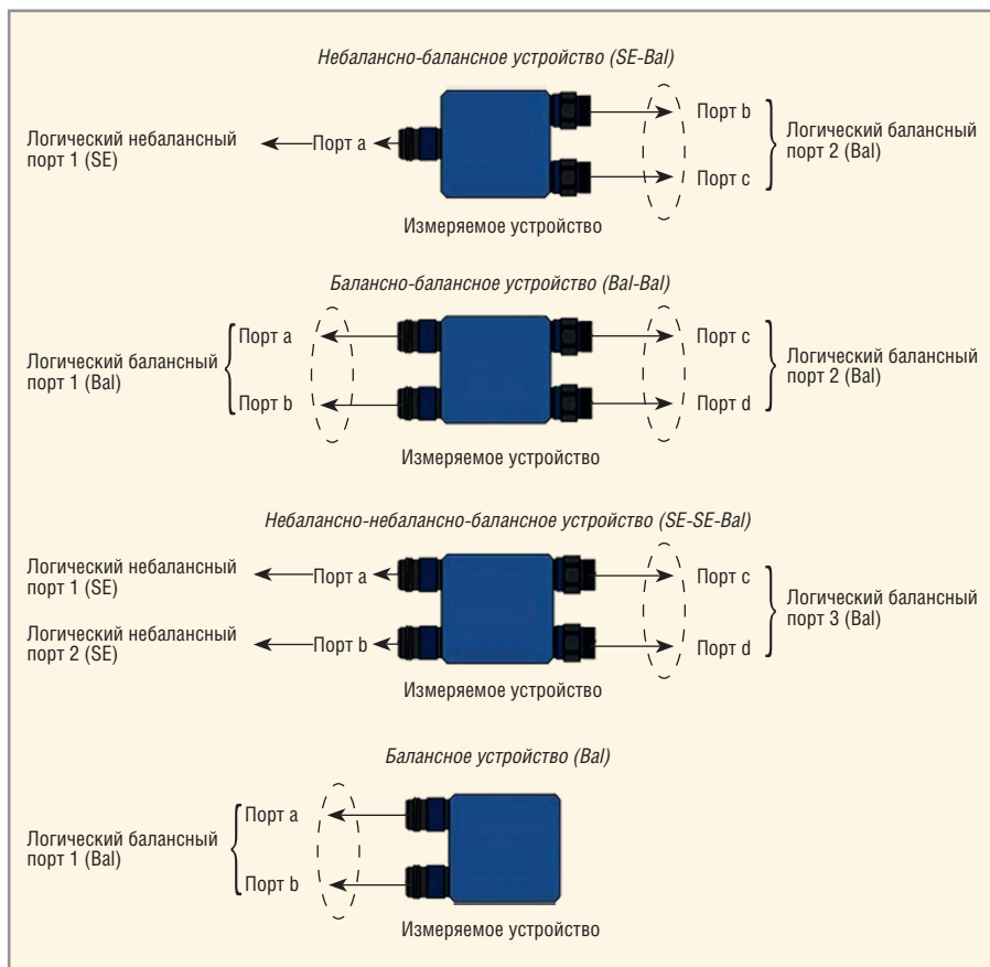
Рис. 5. Типы балансных цепей
