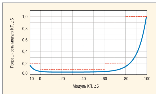
Рис. 9. Погрешность измерений модуля коэффициента передачи
