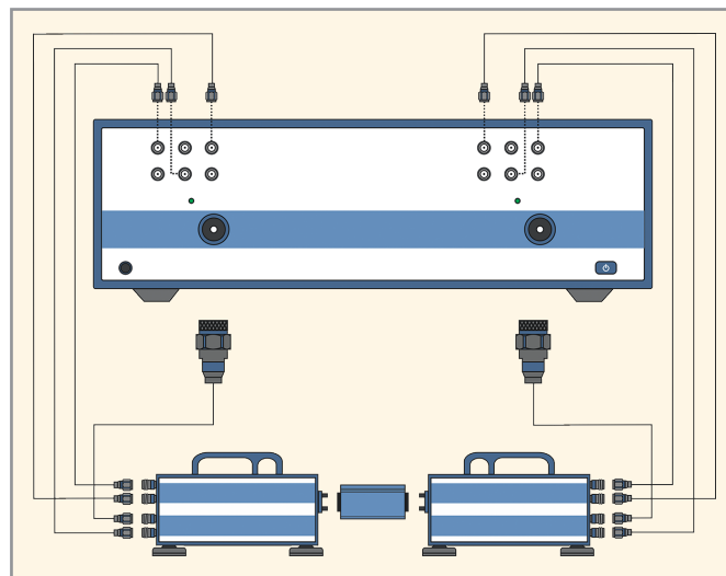
Рис. 4. Измерение S-параметров двухпортового устройства с использованием внешних расширителей
