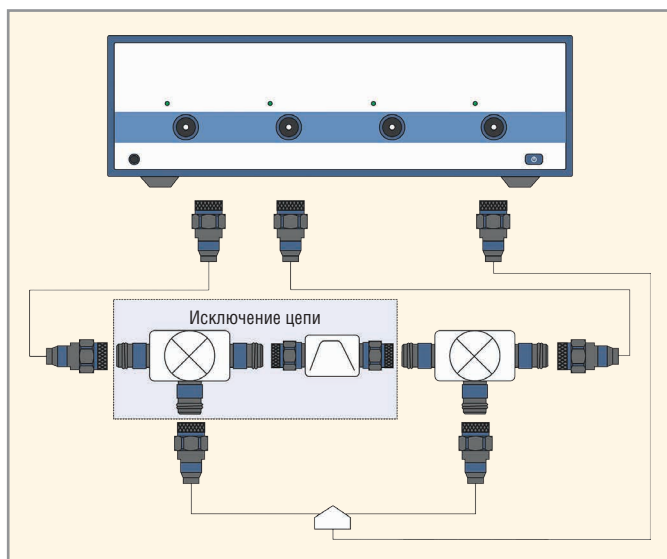
Рис. 6. Измерение параметров смесителя с помощью четырёхпортового прибора
