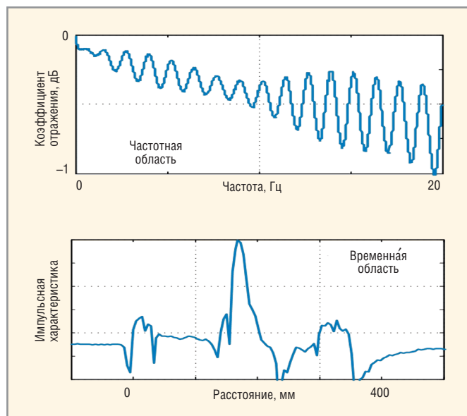
Рис. 7. Расчёт импульсной характеристики цепи
