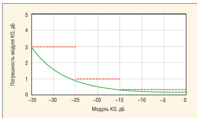
Рис. 8. Погрешность измерений модуля коэффициента отражения
