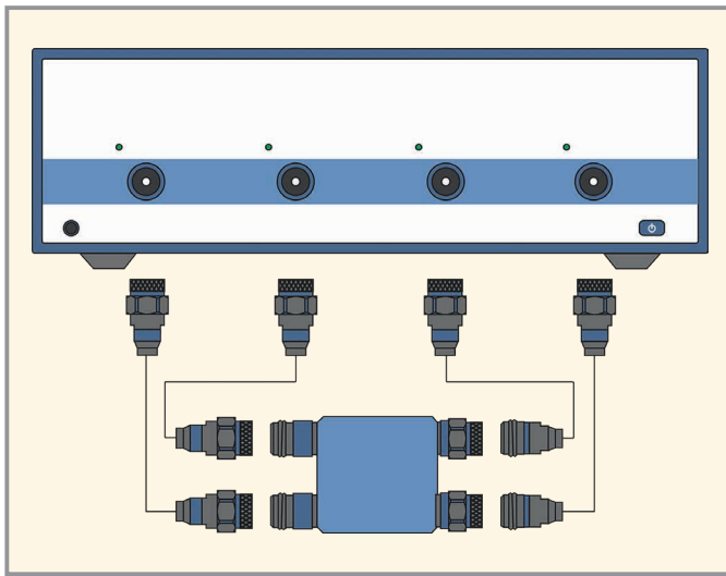
Рис. 1. Одновременное измерение шестнадцати S-параметров четырёхпортового устройства за одно подключение
