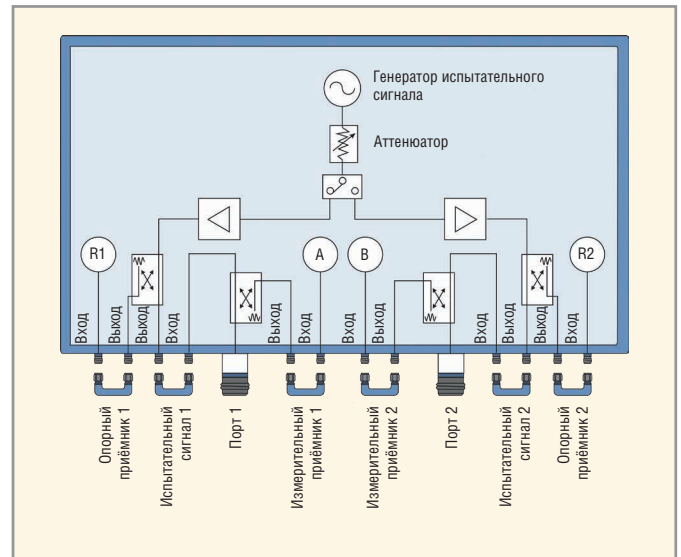
Рис. 2. Расположение перемычек для прямого доступа к приёмникам
