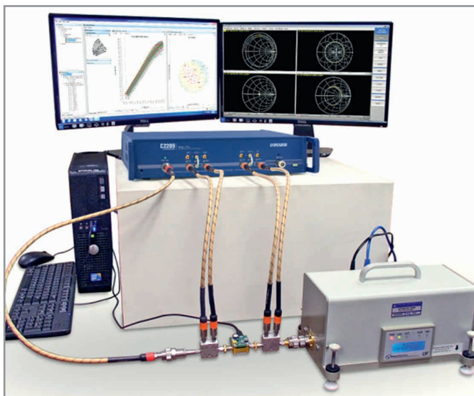
Рис. 3. Измерительная система с переменным импедансом
