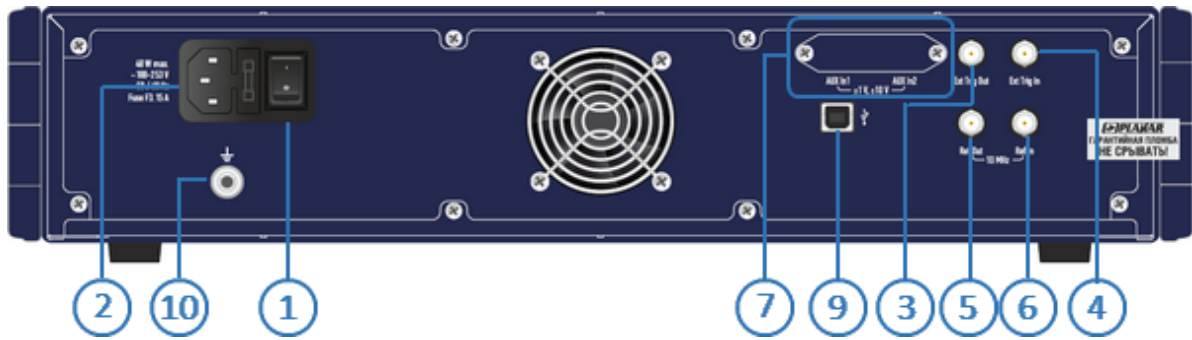
Рисунок 20 – Задняя панель C1409, C2409
