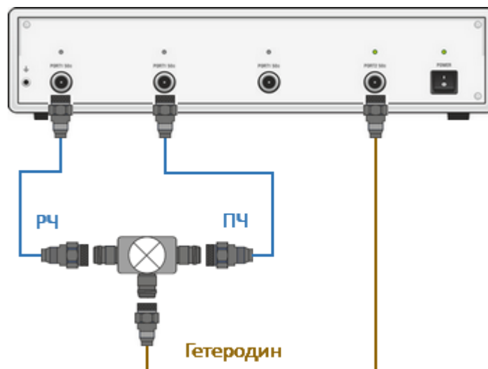
Рисунок 207 – Свободный порт используется как источник сигнала гетеродина
