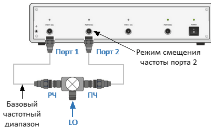
Рисунок 203 – Измерение смесителя с использованием смещения частоты
