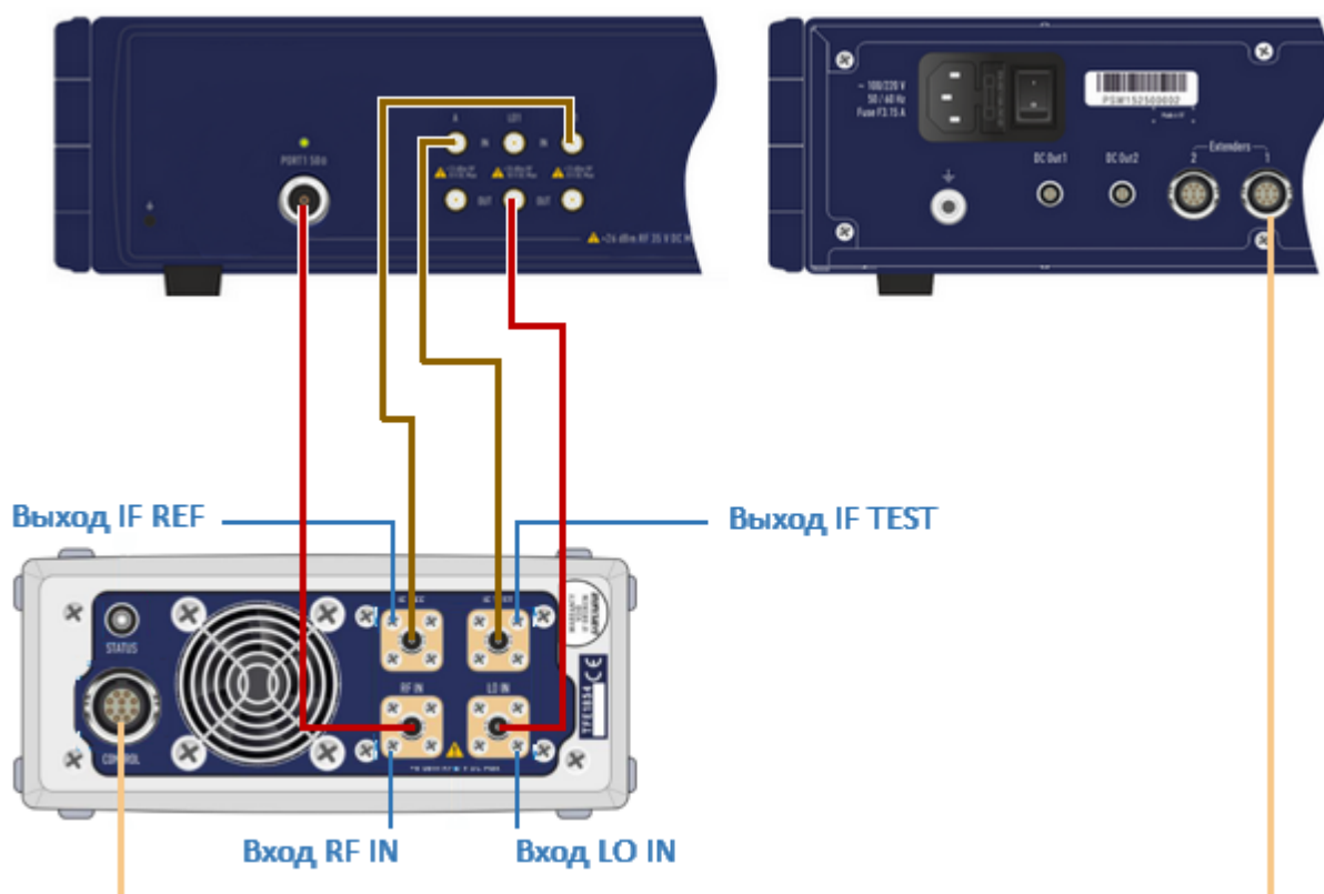
Рисунок 212 – Схема подключения модуля TFE-1854 к анализатору
