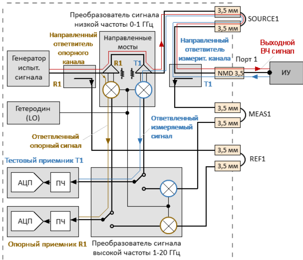
Рисунок 220 – Анализатор С2420, распространение сигнала в общем режиме (диапазон от 100 кГц до 1 ГГц)
