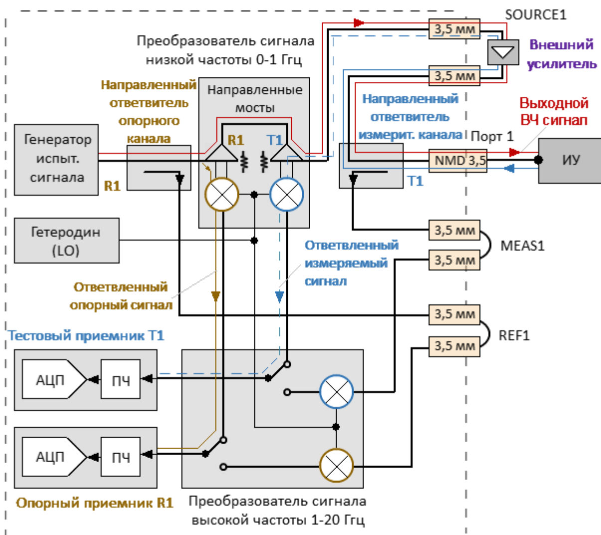
Рисунок 223 – Анализатор C2420, распространение сигнала с внешним усилителем в тракте генератора (диапазон от 100 кГц до 1 ГГц)
