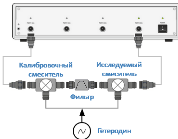
Рисунок 202 – Схема векторного измерения смесителя
