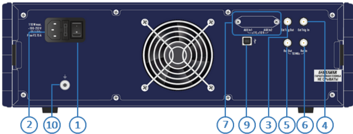
Рисунок 21 – Задняя панель C1420, C2420
