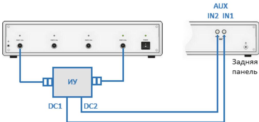
Рисунок 217 – Пример схемы подключения ИУ к вольтметру
