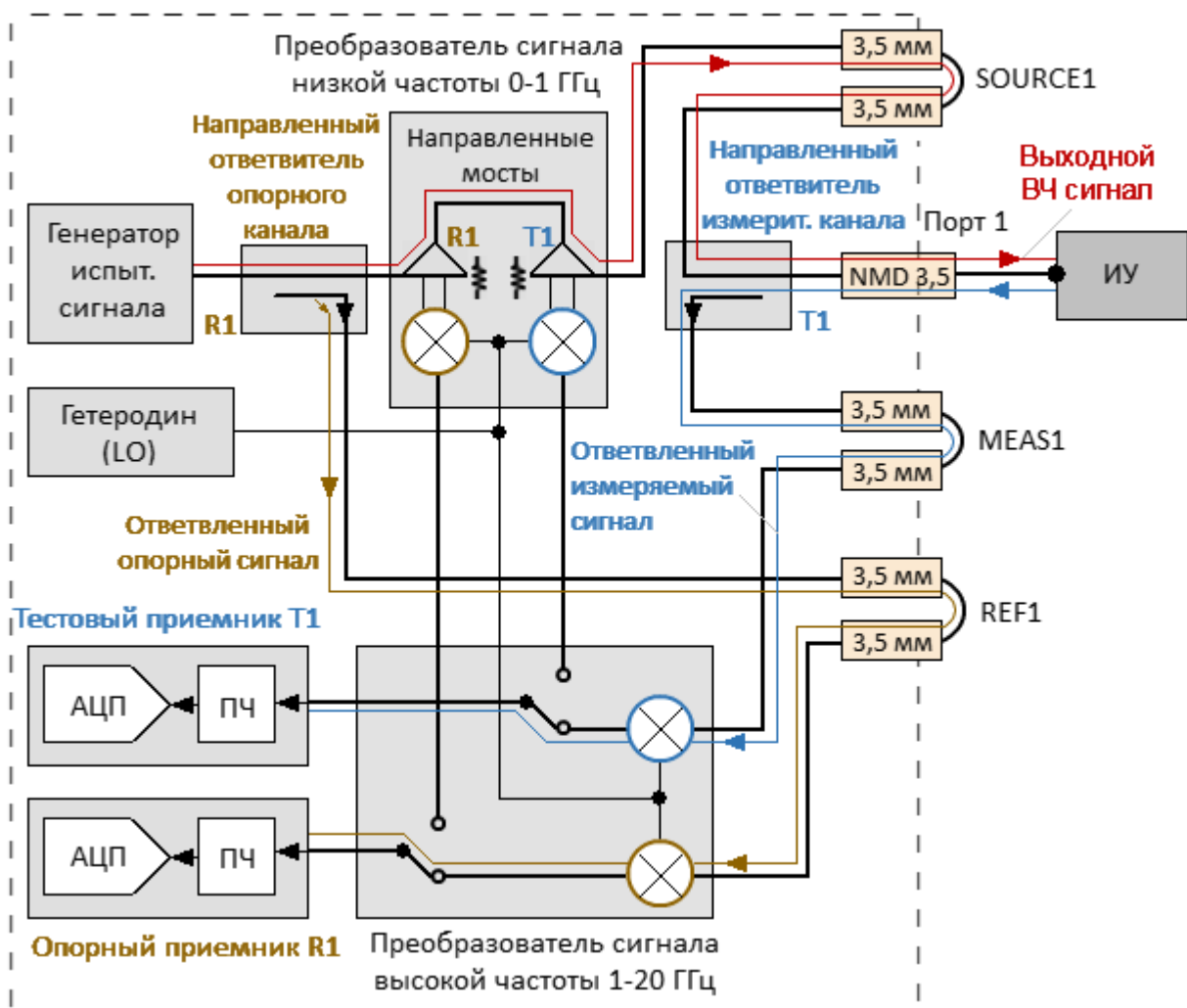
Рисунок 221 – Анализатор С2420, распространение сигнала в общем режиме (диапазон от 1 до 20 ГГц)
