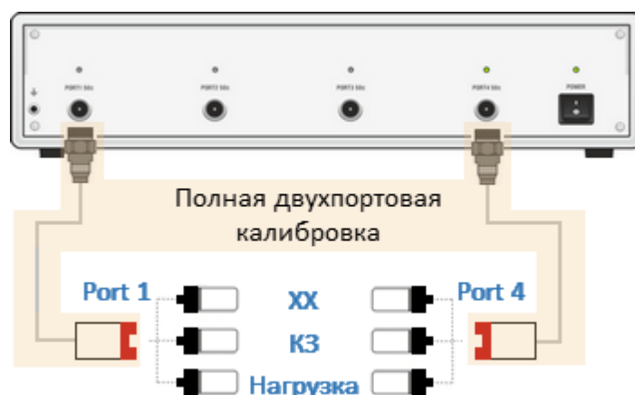
Рисунок 127 – Первый этап калибровки с неизвестной переключкой SOLR
