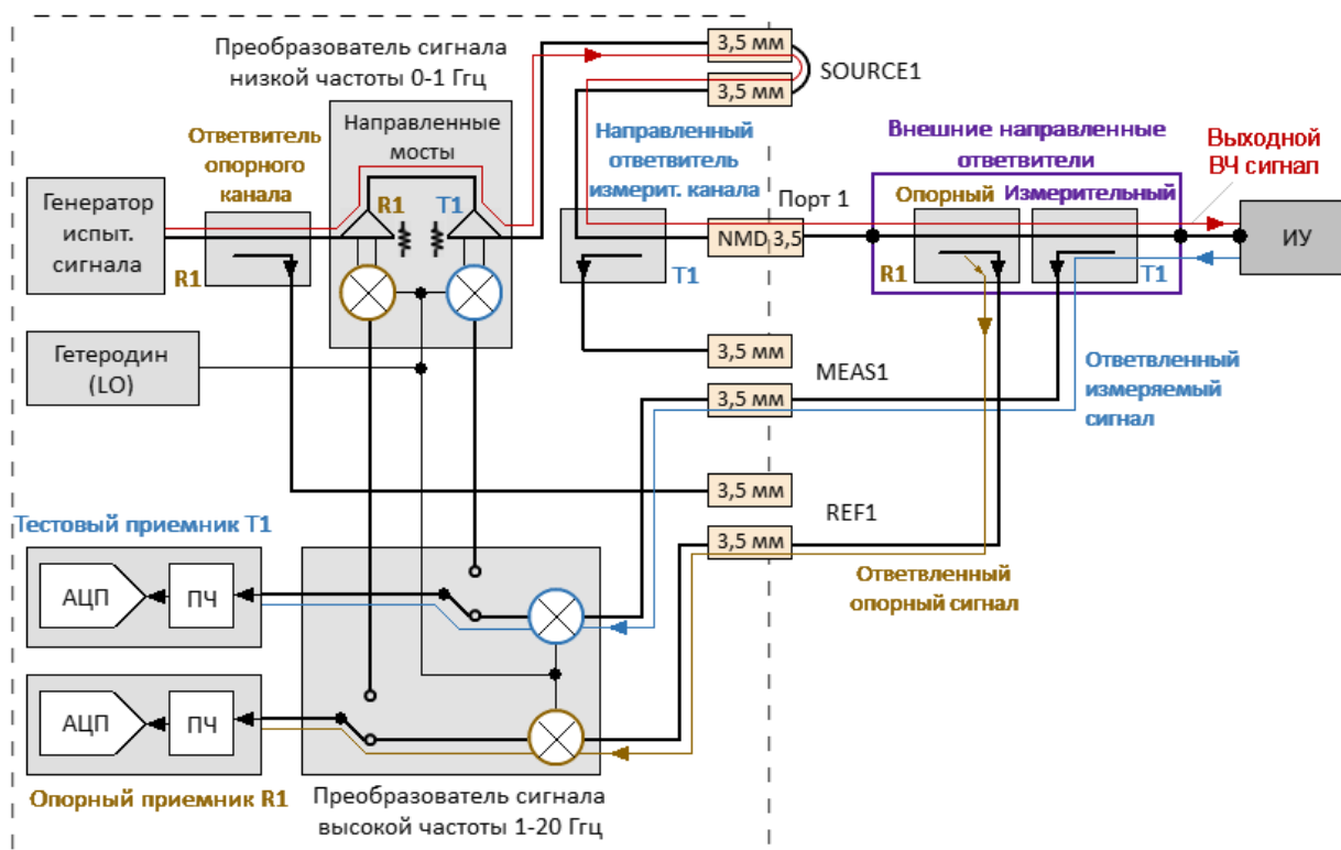
Рисунок 222 – Анализатор C2420, распространение сигнала в режиме прямого доступа
