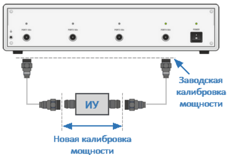
Рисунок 138 – Калибровка мощности
