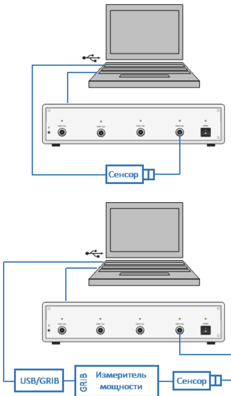
Рисунок 224 – Пример подключения измерителя мощности
