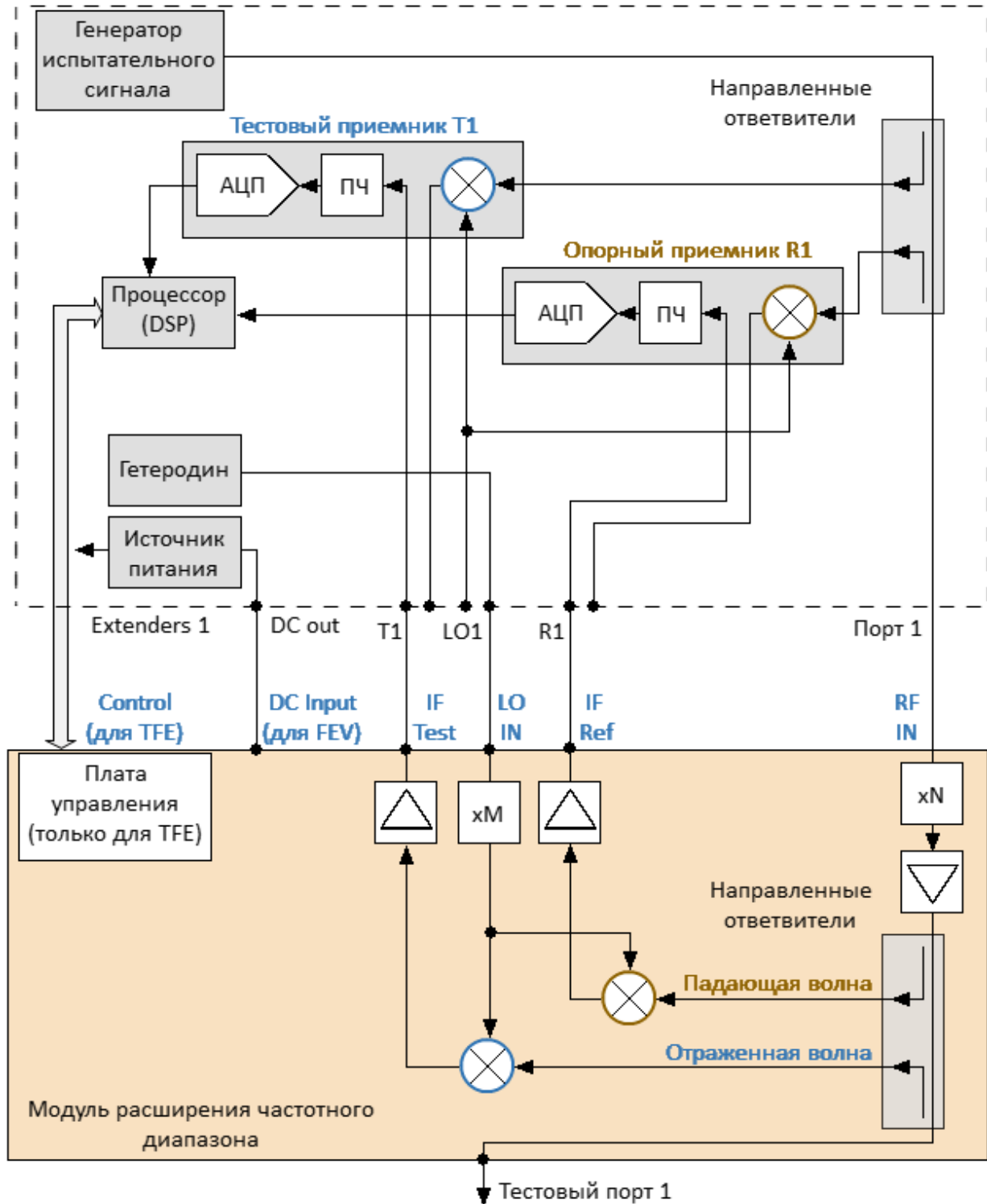
Рисунок 208 – Структурная схема подключения модуля к анализатору
