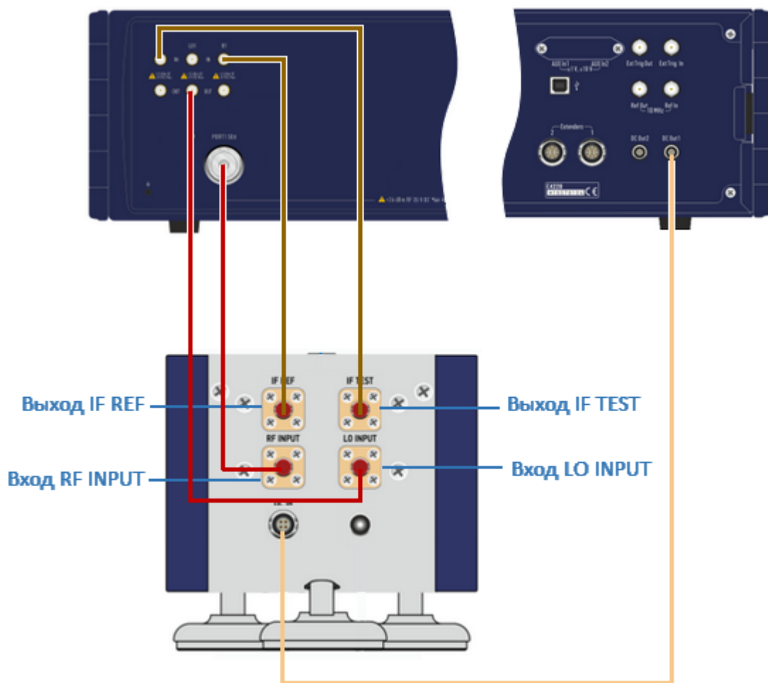
Рисунок 214 – Схема подключения модуля FEV к анализатору
