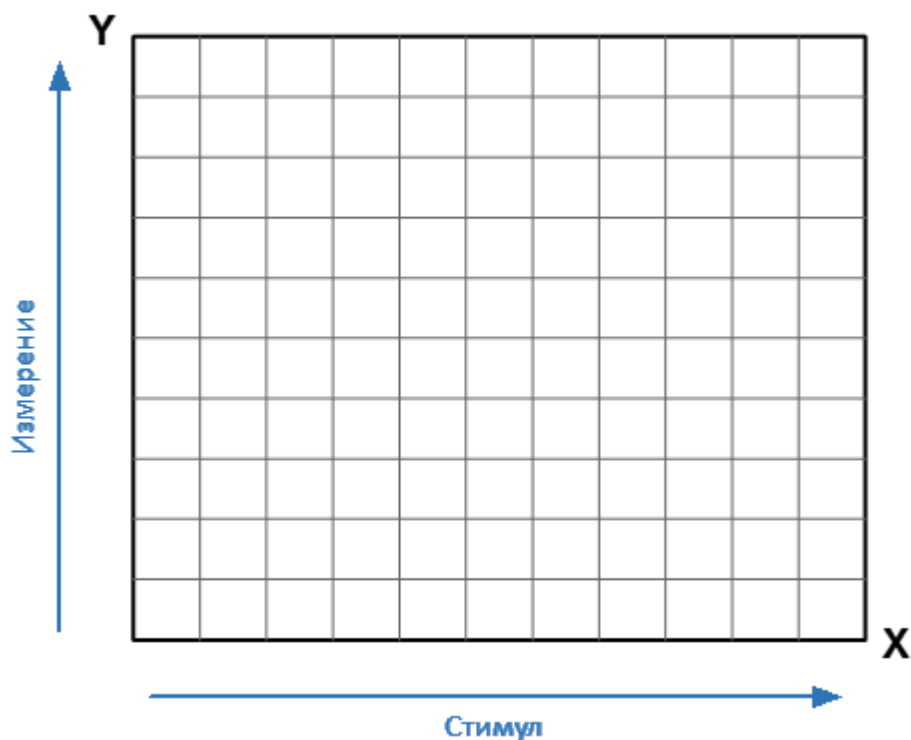
Рисунок 59 — Прямоугольные координаты
