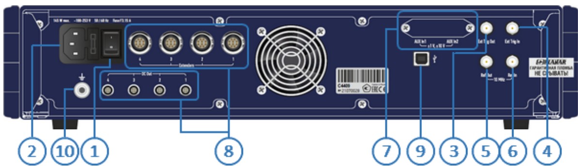
Рисунок 22 – Задняя панель C4409
