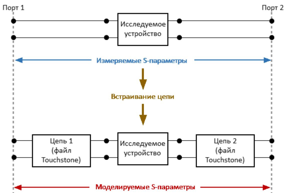
Рисунок 182 – Встраивание цепи
