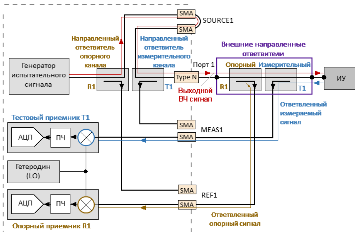
Рисунок 219 – Анализатор С2409, распространение сигнала в режиме прямого доступа
