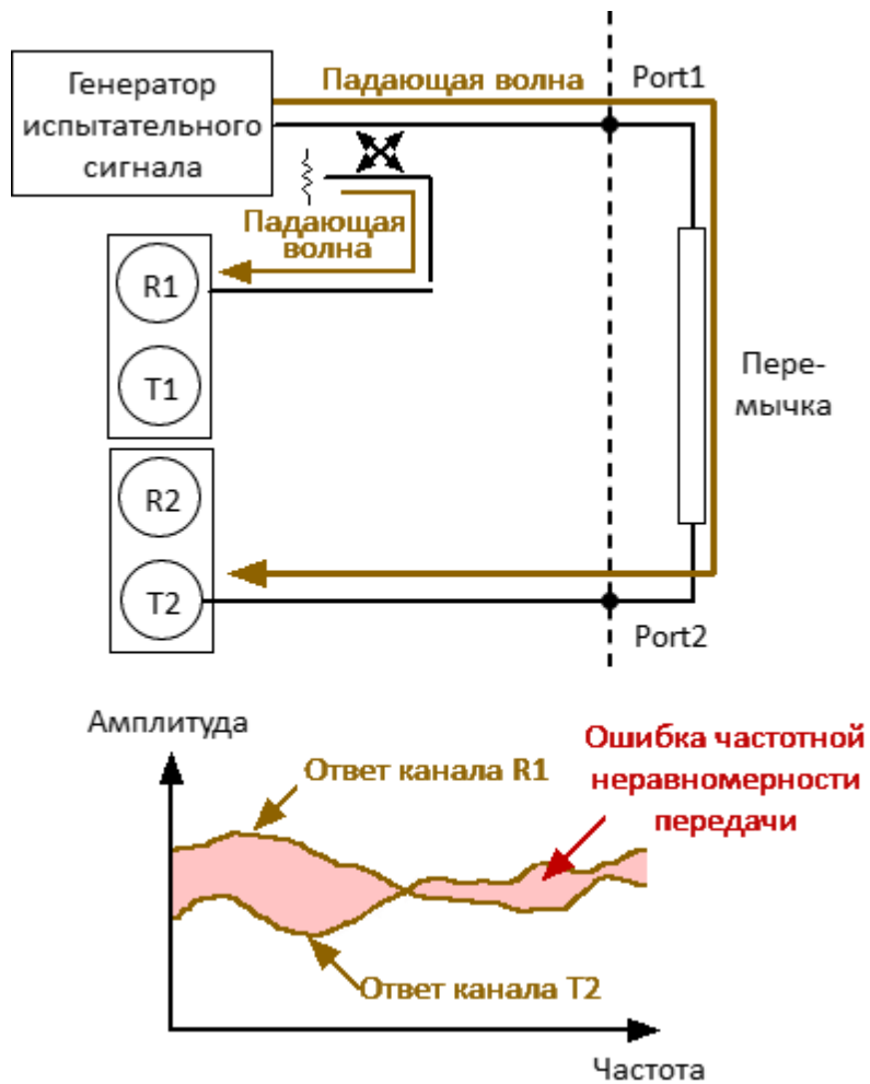
Рисунок 101 – Ошибка частотной неравномерности передачи
