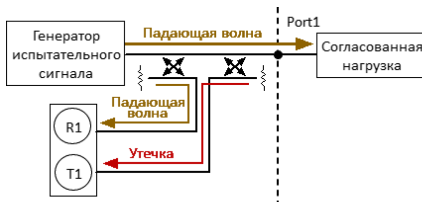
Рисунок 97 – Ошибка направленности
