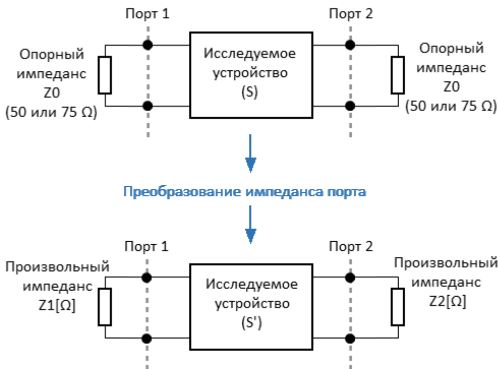
Рисунок 180 – Преобразование импеданса порта
