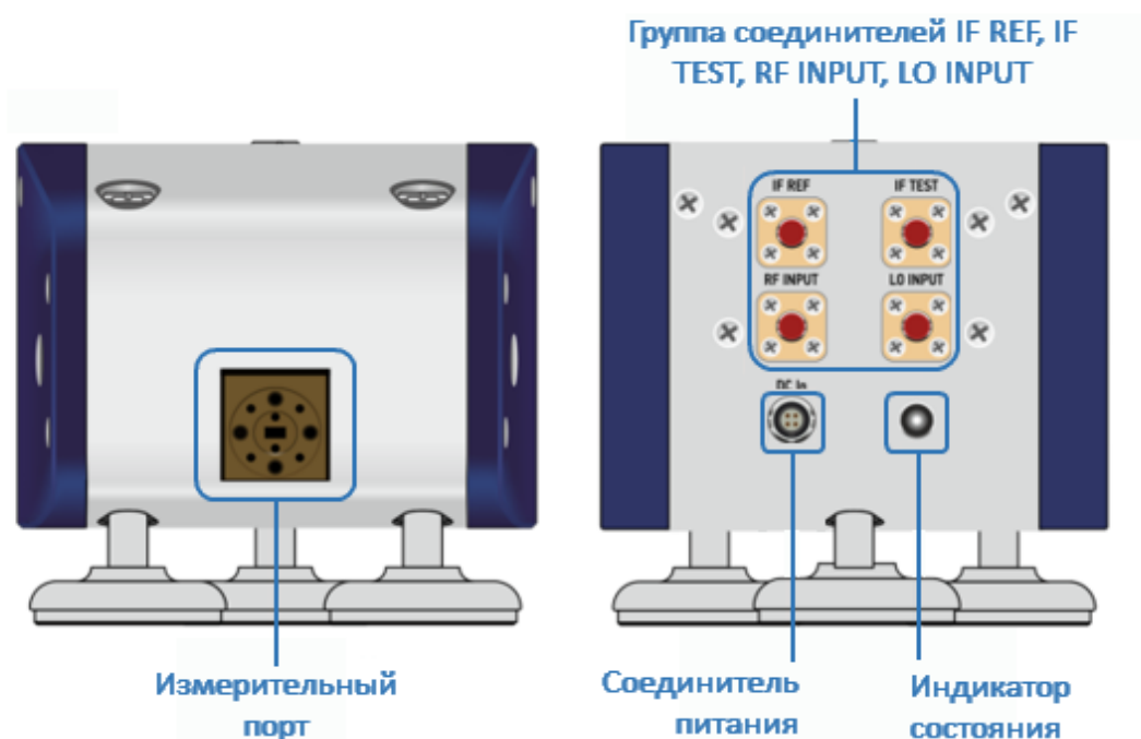
Рисунок 213 – Передняя и задняя панели модуля FEV
