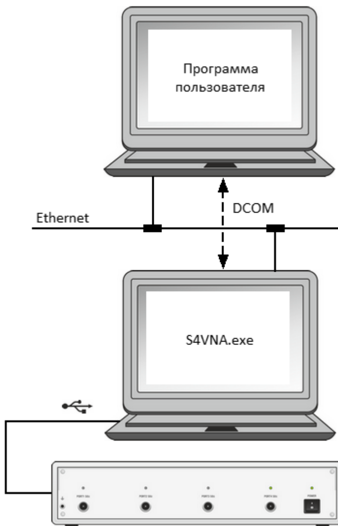
Рисунок 243 – Технология DCOM
