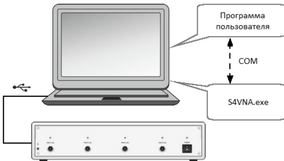
Рисунок 242 – Технология COM
