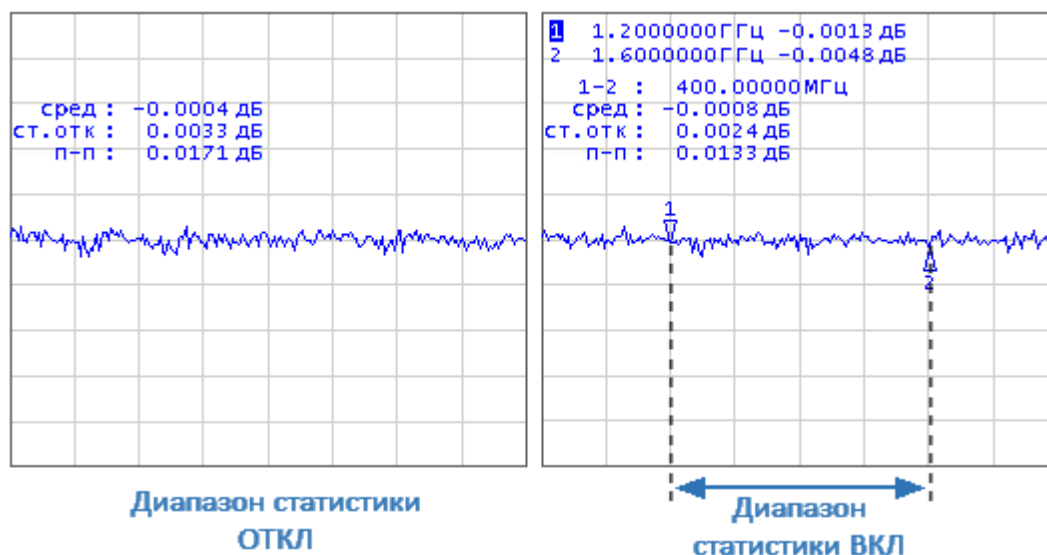
Рисунок 171 – Статистика
