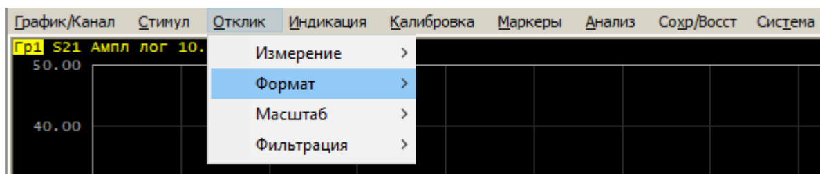
Рисунок 34 – Строка меню
