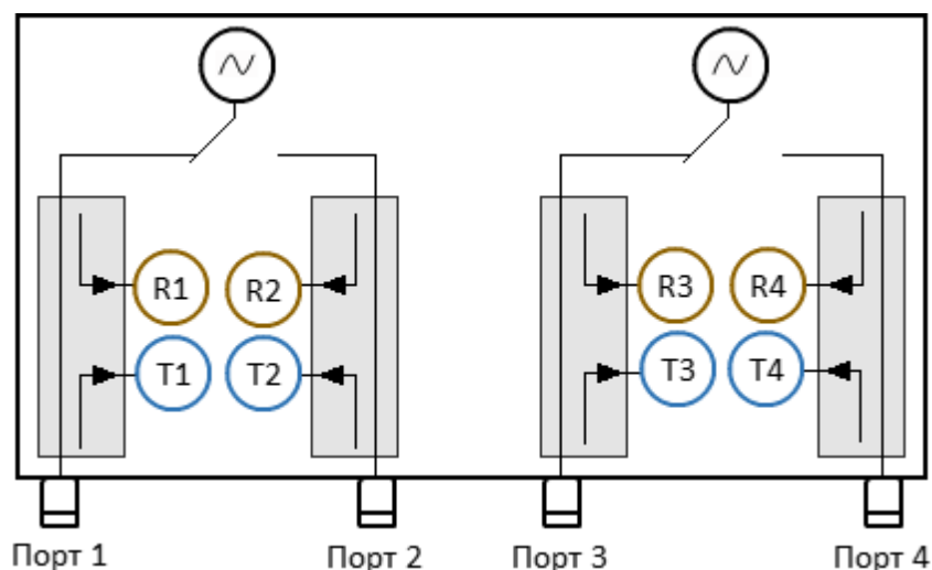
Рисунок 206 – Структурная схема четырехпортового анализатора
