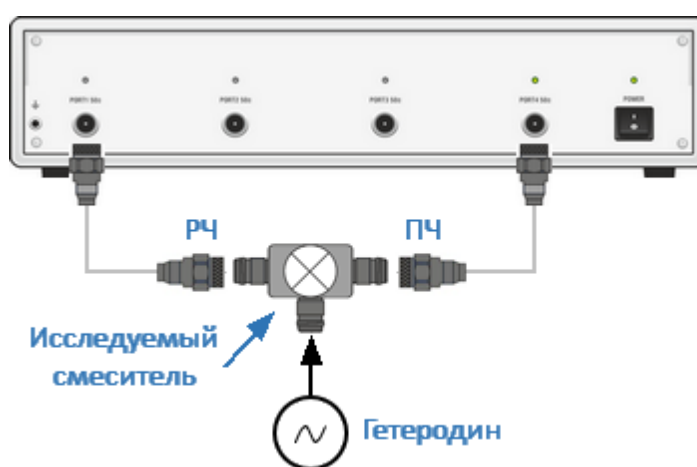
Рисунок 201 – Схема скалярного измерения смесителя
