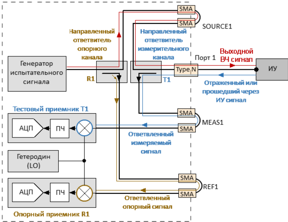
Рисунок 218 – Анализатор C2409, распространение сигнала в общем режиме
